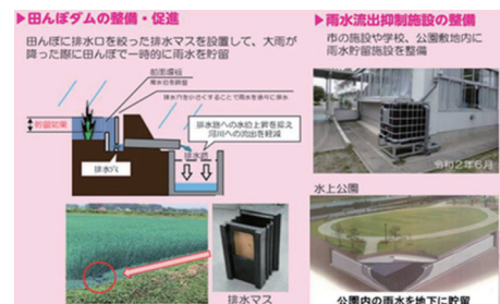
図2 流域治水を推進させる宇都宮市の取組
